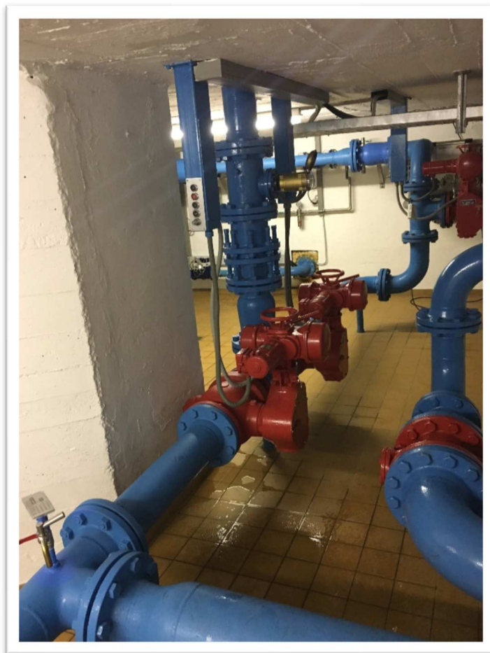
Bild 6: Ansicht in den Rohrkeller mit beengten Verhältnissen unterhalb des Aufstellortes der Reinwasserförderpumpen
