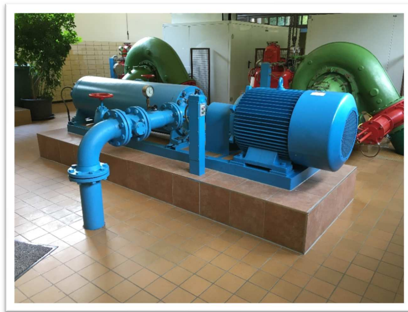
Bild 5: Ansicht auf die bestehende Reinwasserförderpumpe
